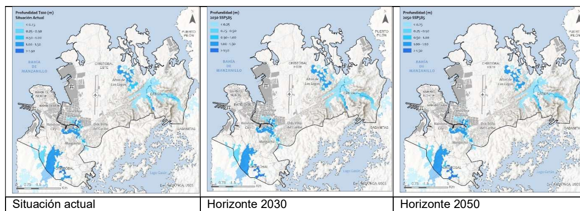
Figura 14 – Mapas de profundidad de la lámina de agua para el evento de 100 años de periodo de retorno en la situación actual y los horizontes 2030 y 2050 SSP585.
