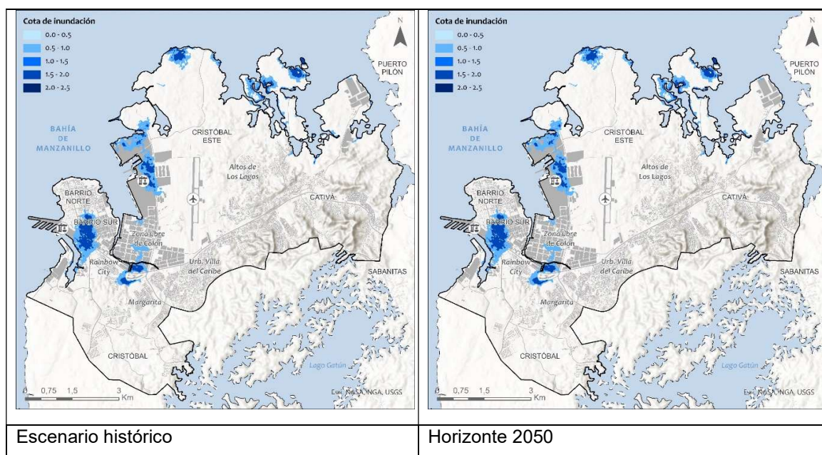
Figura 15 – Mapas del impacto de inundación costera para un evento extremo de 100 años de periodo de retorno en el escenario histórico y (percentil del 95%) en el horizonte 2050 para el escenario de emisiones SSP5-8.5.
