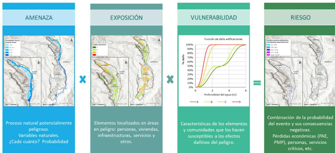
Figura 13 – Esquema amenaza-exposición-vulnerabilidad-riesgo
